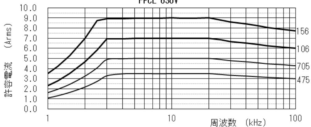
周波数別許容実効電流 FPCL 630V
