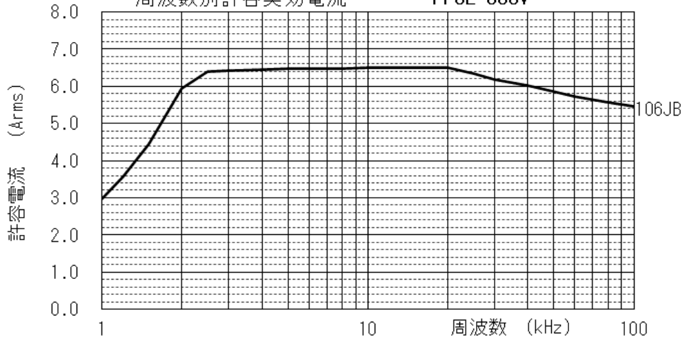
周波数別許容実効電流 FPCL 800V
